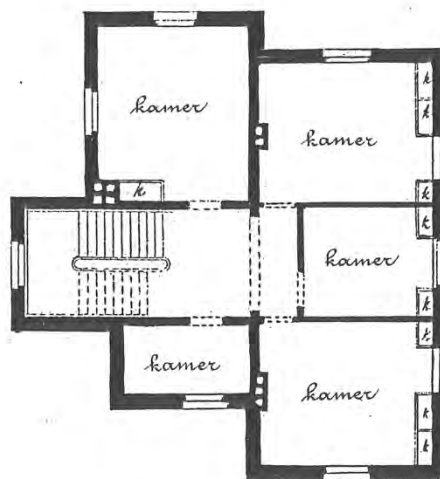
Bovenverdieping.
