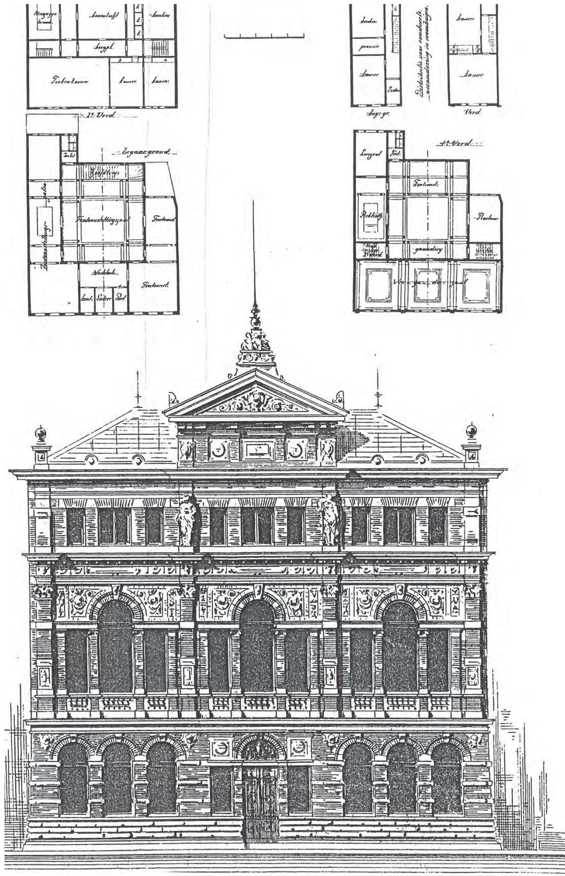
4. Gebouw voor permanente tentoonstellingen, 1885. ( Bouwkundig weekblad 1885, 205)
