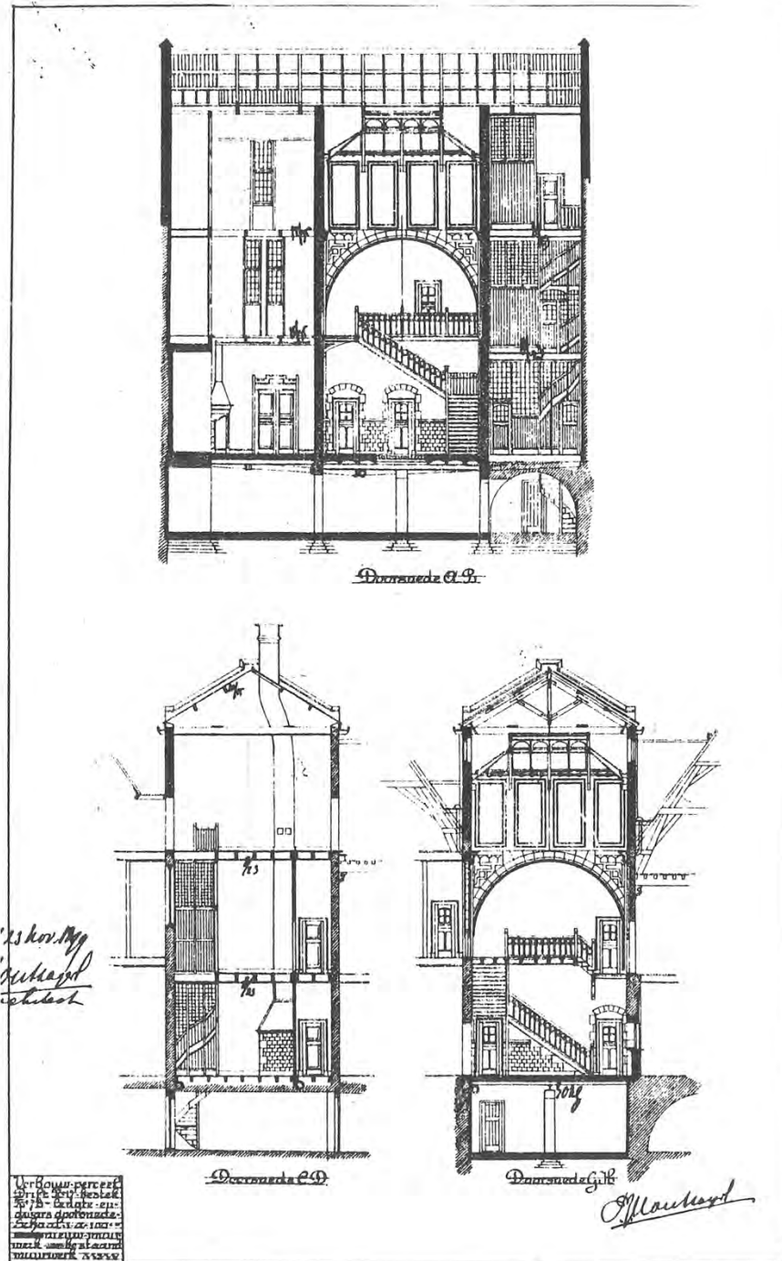
59. Idem 58, doorsneden. (V.B., GAU)
