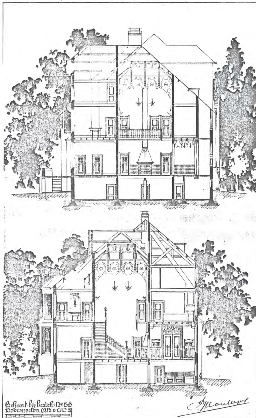
VILLA-ONTWERP „HUIS TER HEIDE“ AAN DEN STRAATWEG UTRECHT--SOESTERBERG. * F. J. HOUTZAGERS (UTRECHT) ARCH. *
