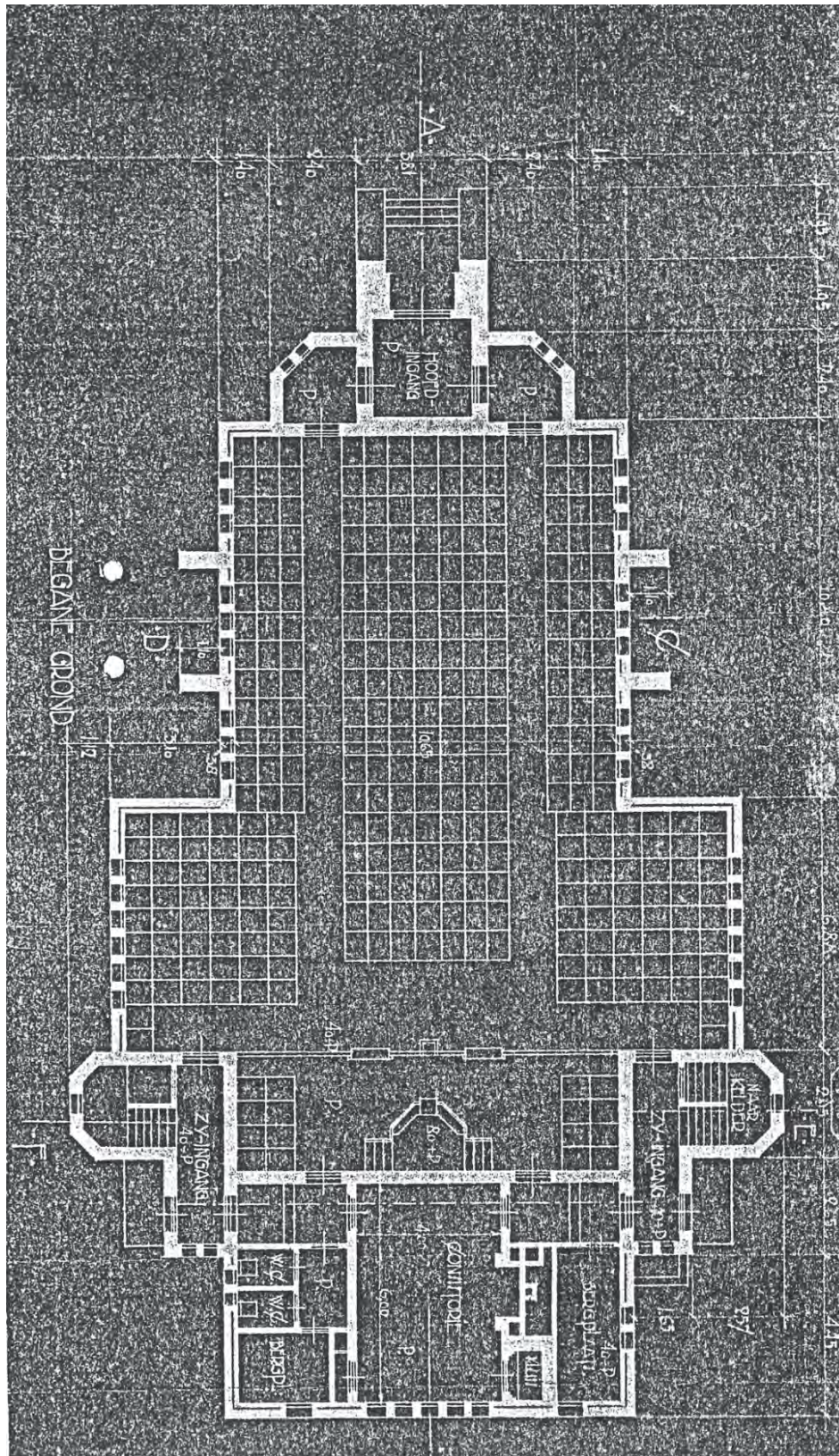
85. Gereformeerde kerk Soestdijkseweg, De Bilt, 1922. Plattegrond. (V.B. gemeente De Bilt.)
