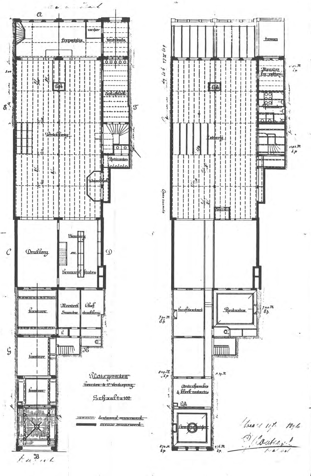
40. Idem 39, plattegronden. (V.B., GAU)
